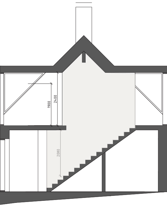
SEKTION C
