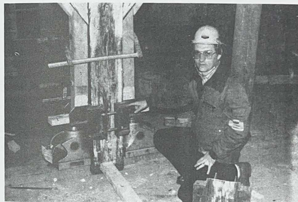
Övre bilden visar hur de rötskadade bjälklagen reparerades. Undre hur avvägningen av bjälklagen gjordes.
